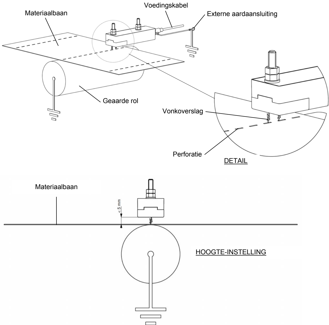
Afbeelding 3, installatie Perfomaster
