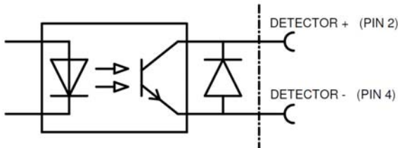
Afbeelding 4, aansluitingen Perfomaster
