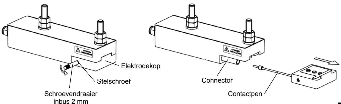
Afbeelding 6, vervangen elektrodekop
