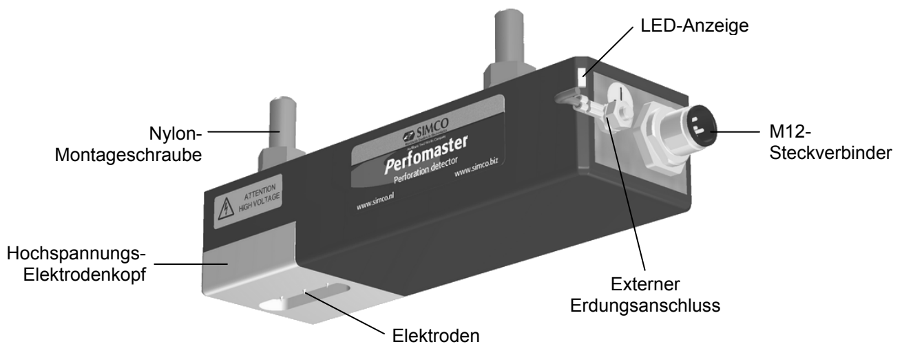
Abbildung 1, Perfomaster
