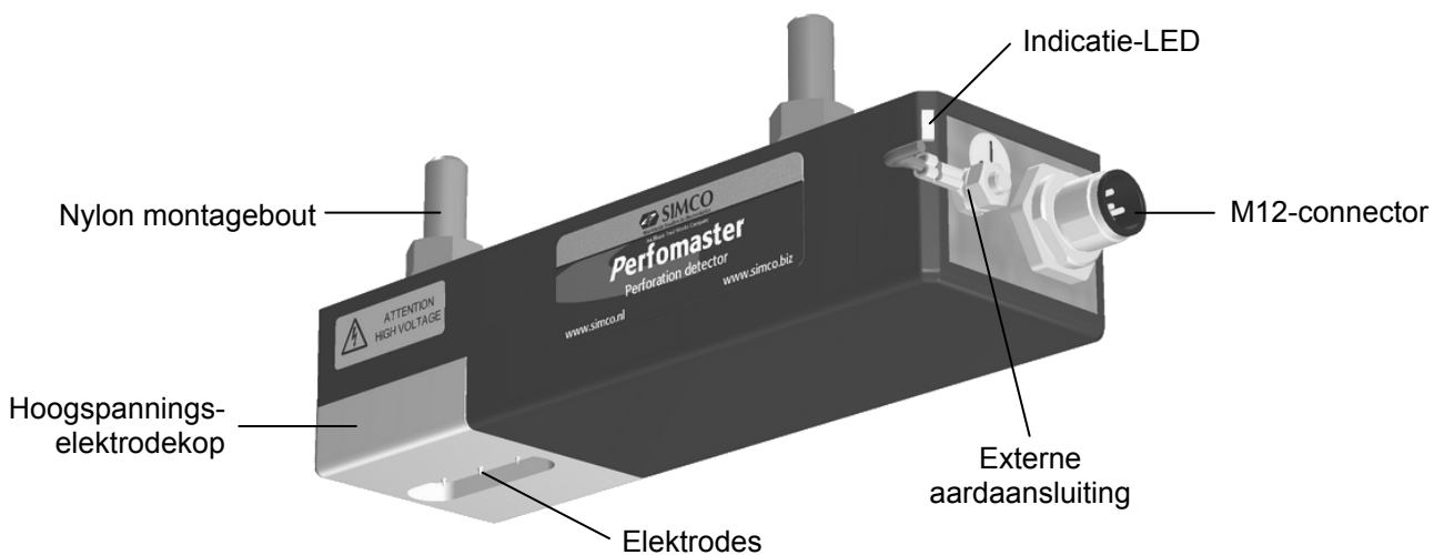
Afbeelding 1, Perfomaster
