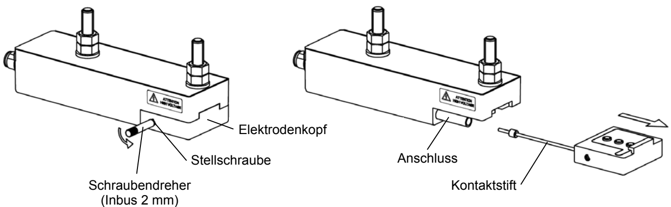
Abbildung 6, Elektrodenkopf ersetzen
