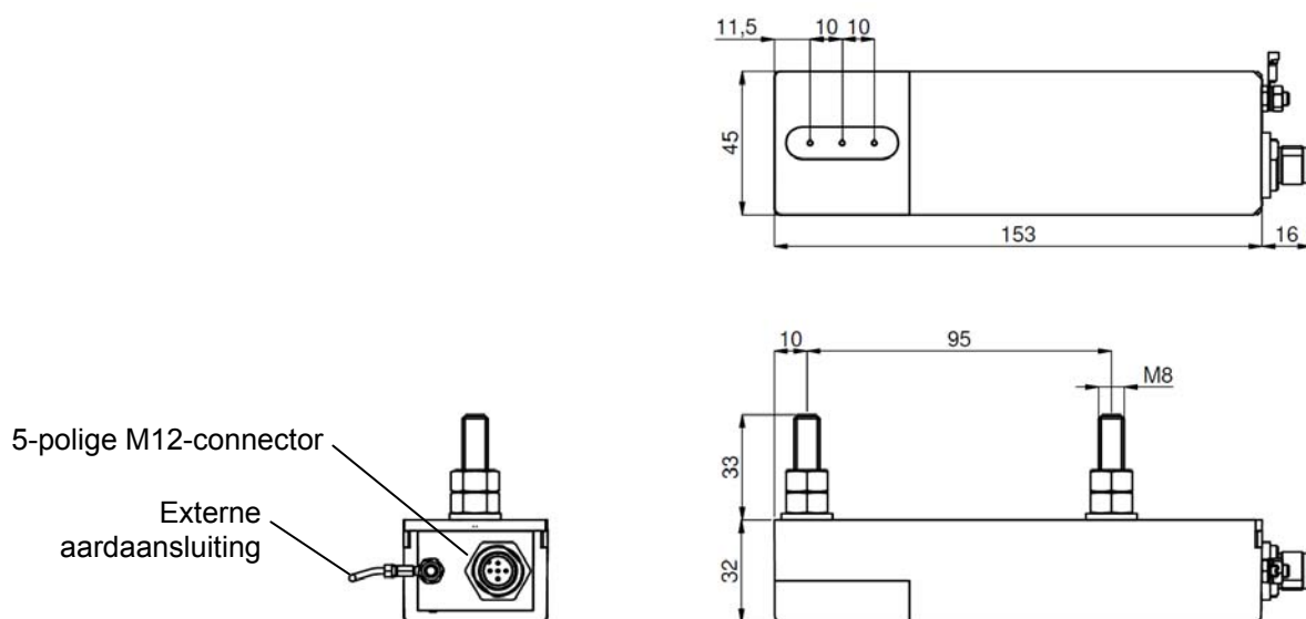
Afbeelding 2, afmetingen Perfomaster
