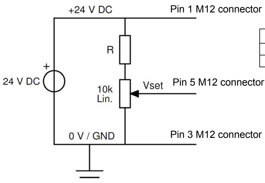
Afbeelding 5b, voorbeeldschema voor aanbieden instelspanning d.m.v. weerstandsdeling van voedingsspanning (Application Note)
