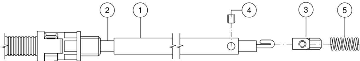
Afbeelding 2: montage HV-connector
