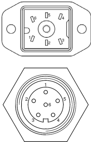
Fig. 1 Lay out 6-polige connectoren: Control Module + Thunder/ON (voor-aanzicht chassisdelen).
