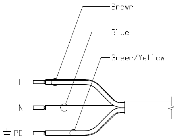
Fig. 2 Aansluiten netsnoer
